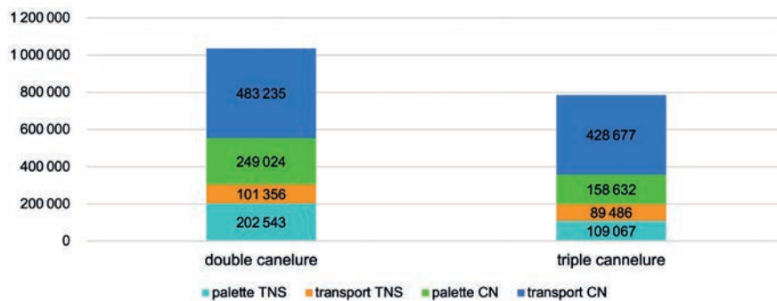
Baisse d'impact transport lié à l'optimisation de palettisation (kg eqCO 2 , pour deux millions de produits ; fabrication répartie 50/50 entre Tunisie et Chine)
