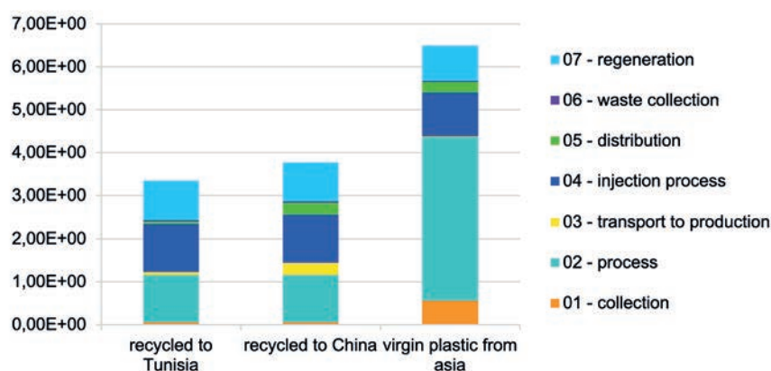
Comparaison des impacts entre le plastique vierge et recyclé, en fonction du lieu de fabrication des produits finis (Kg eq. CO2 / kilo de plastique)
