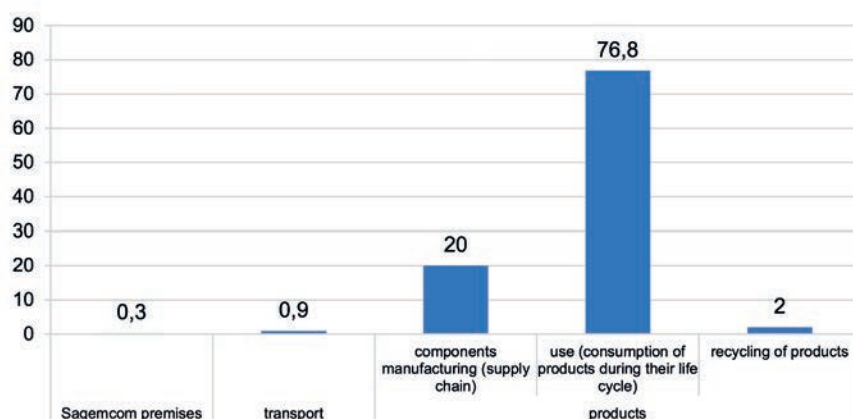
Répartition de l'impact carbone annuel de Sagemcom
